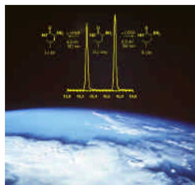
La figure illustre la formation de Leucine asymétrique dans l'espace interstellaire. Le fond de l'image a été adapté d'après une photo prise en juin 1988 par l'équipage STS-91 de la navette spatiale Discovery
