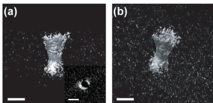
FIGURE 1.15 – Reconstitution par tomographie d'un nanopore sur support silicium [44]. Les barres d'échelle indiquent 5 nm.
