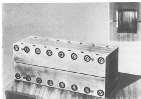
FIG. 2.3: Polarisation d'un faisceau de neutrons : a) Principe de la polarisation en spin d'un faisceau de neutrons : un faisceau de neutrons non polarisés (c'est-à-dire où la moitié des neutrons sont dans l'état de spin |+\rangle et l'autre moitié dans l'état |-\rangle ) interagit avec une structure ferromagnétique pour laquelle b_N = \gamma r_0 f_a(\mathbf{Q})M (où b_N = -\gamma r_0 f_a(\mathbf{Q})M ). Seuls les neutrons polarisés |+\rangle (ou |-\rangle ) sont diffusés b) Monochromateur double focalisant de Heusler constitué de 65 monocristaux de Heusler produits par l'ILL. c) Vue d'un bender formé de plusieurs dizaines de supermiroirs de CoFe/TiGd
