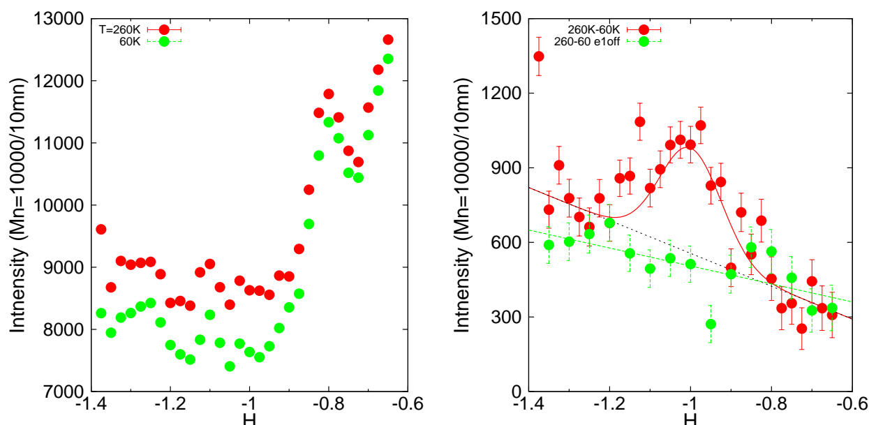
FIG. 6.10: Etude sur 3T1 du composé \text{La}_{2-x}\text{Sr}_x\text{CuO}_4 a) Coupe le long de la direction (H,0,L) autour de H=-1 pour T=260\text{K} (points rouges) et T=60\text{K} (points verts). Pour chacune des ces valeurs, on ajuste la valeur de L pour que k_f soit parallèle à la direction (0,0,L) . b) Différence entre T=260\text{K} et 60\text{K} le long de la direction (H,0) en mode intégration. Les points rouges correspondent à la différence entre les données présentées en a). En points verts : même chose pour l'échantillon désaligné (de 10^\circ ), |Q| reste constant mais la direction de Q a changé. On représente en ligne rouge l'ajustement gaussien des points rouges. On déduit de l'ajustement que l'intensité du pic est de 430cts (en 588s) avec une largeur \Delta H=0.2 r.l.u. Il est intéressant de noter que la largeur du pic est très proche de la largeur du pic statique reportée dans la partie 6.2.3.
