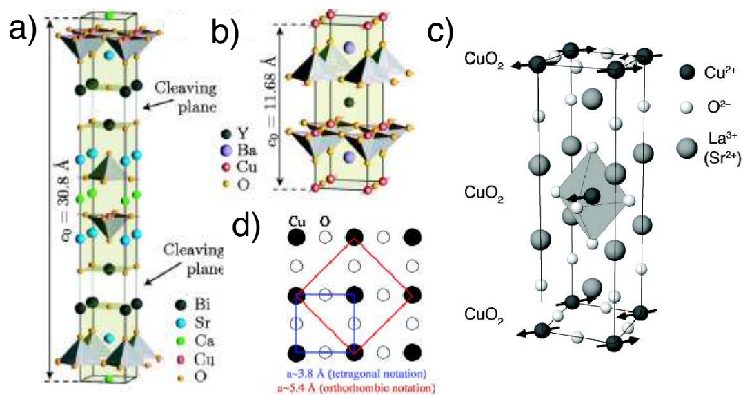
FIG. 2.6: Structure cristallographique des trois SHTCs étudiés durant cette thèse : a) \text{Bi}_2\text{Sr}_2\text{CaCu}_2\text{O}_{8+x} b) \text{YBa}_2\text{CuO}_{6+x} et c) \text{La}_{2-x}\text{Sr}_x\text{CuO}_4 (les flèches correspondent à l'ordre AF des spins du cuivre dans le cas non dopé ( x=0 )). Sur ces trois figures, on a mis en évidence l'octaèdre \text{CuO}_6 . d) Différentes descriptions du plan \text{CuO}_2 : la cellule élémentaire en notation orthorhombique est représentée en rouge, la cellule élémentaire en notation tétragonale est représentée en bleu (en notation orthorhombique, la cellule élémentaire est deux fois plus grande et tournée à 45^\circ de la cellule élémentaire en notation tétragonale)
