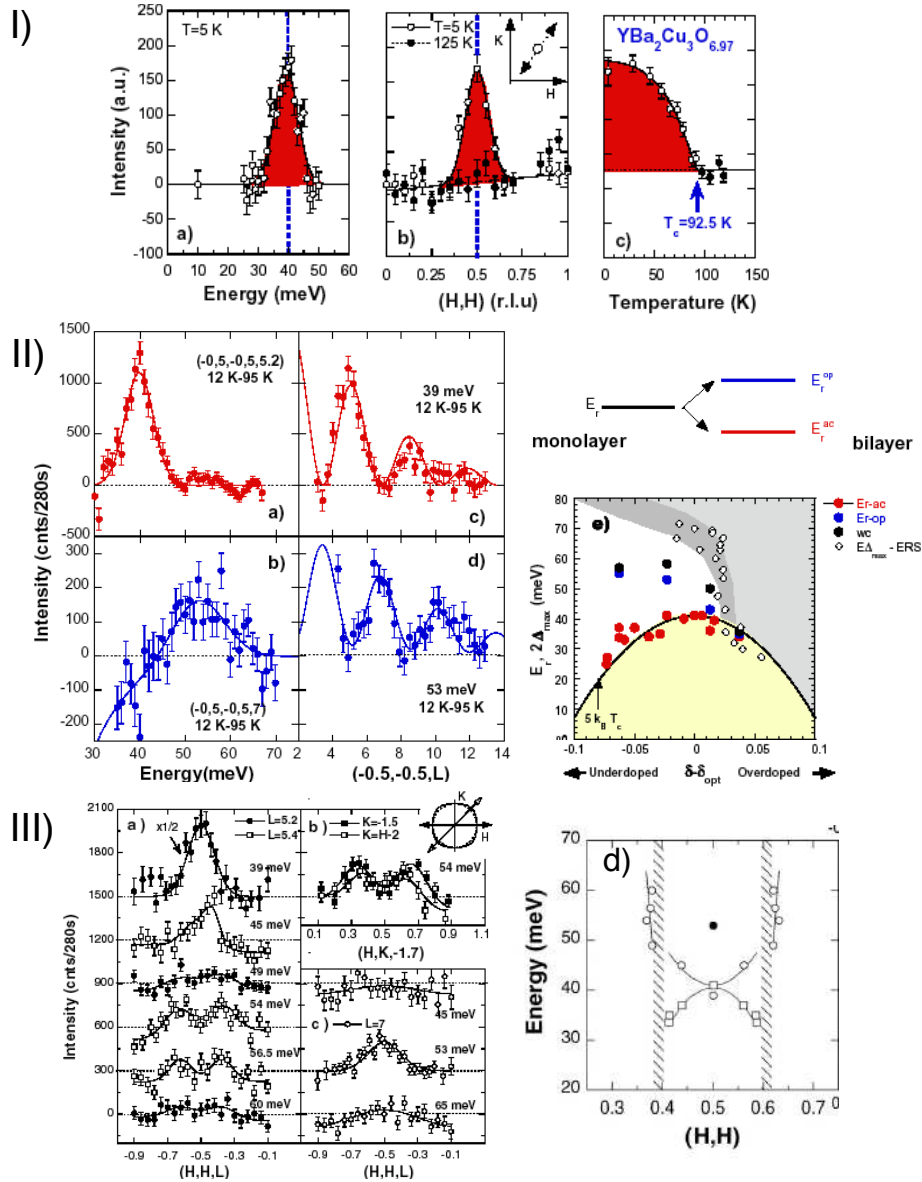
FIG. 1.7: I) Présentation du pic de résonance magnétique mesuré dans le composé \text{YBa}_2\text{Cu}_3\text{O}_{6.97} de T_c = 92.5 \text{ K} par DIN : a) Intensité mesurée à basse température T = 5 \text{ K} en fonction de l'énergie au vecteur d'onde AF, b) Intensité le long de la direction (H,H) pour une énergie de 41 meV à basse (point blanc) et haute température (point noir) c) Evolution en température mesurée aux vecteurs d'ondes Q = (0.5, 0.5, 4.7) pour une énergie de 41 meV. II) Différence entre les scans au vecteur d'onde AF à basse température et juste au dessus de T_c pour un échantillon \text{YBa}_2\text{Cu}_3\text{O}_{6.85} de T_c = 89 \text{ K} a) et c) Pics de résonance magnétique dans le canal acoustique avec sa modulation typique en sinus carré b) et d) Même chose dans le canal optique. e) Dépendance en dopage de l'énergie caractéristique du mode acoustique (en rouge) et du mode optique (en bleu). Les deux modes se trouvent en dessous de 2\Delta_m qui représente l'énergie minimum pour créer une excitation élémentaire au vecteur d'onde AF. 2\Delta_m peut être mesuré par ARPES, SIS ou encore Raman. III) Différence d'intensité entre basse température ( T = 10 \text{ K} ) et T_c plus 10 K dans un échantillon \text{YBa}_2\text{Cu}_3\text{O}_{6.85} de T_c = 89 \text{ K} , le long de la direction (H,H) pour différentes énergies a) L = 5.2 ou 5.4 (canal acoustique) c) L = 7 (canal optique) et b) coupe à énergie constante pour deux directions de l'espace réciproque (1,0,0) et (1,1,0) d) Dispersion des excitations magnétiques dans la phase supraconductrice déduite des mesures reportées en a).
