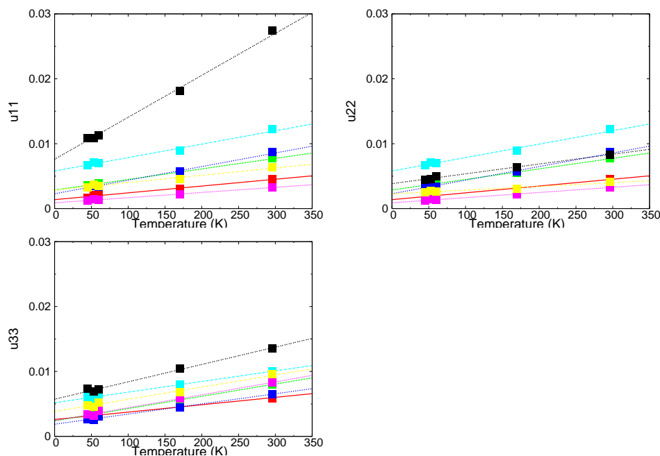
FIG. A.3: Déplacement moyen des atomes de la maille YBCO6.5 le long des trois directions ( a^* , b^* , c^* ) en fonction de la température. Les lignes correspondent à l'ajustement linéaire réalisé pour chacun des atomes
