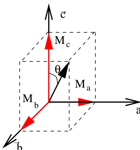
FIG. 5.6: Schéma représentant l'orientation du moment M. L'angle \theta correspond à l'angle entre le moment M et l'axe cristallographique c. Dans le cas de la phase CC-\theta_{II} , on attend \theta = 0^\circ
