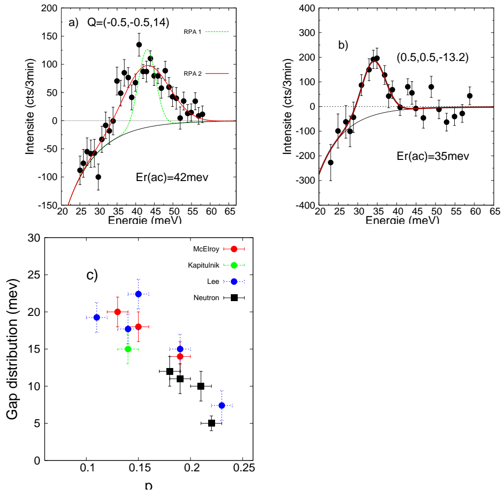
FIG. 3.15: a) et b) Résonance magnétique pour Bi-2212 T_c=87\text{K} et 70\text{K} mesurée à Q=(-0.5,-0.5,14) et Q=(0.5,0.5,-13.2) . Les lignes pleines correspondent à la susceptibilité magnétique déduite par RPA convoluée avec la fonction de résolution : en vert on représente le cas d'un gap de symétrie d (RPA 1) et en rouge on représente le cas d'une distribution de gap de symétrie d (RPA 2) c) Largeur à mi-hauteur de la distribution de gap mesurée par STM [183, 173, 182] et largeur du pic de résonance magnétique déconvoluée de la résolution expérimentale, mesurée par DIN[99, 177, 157].
