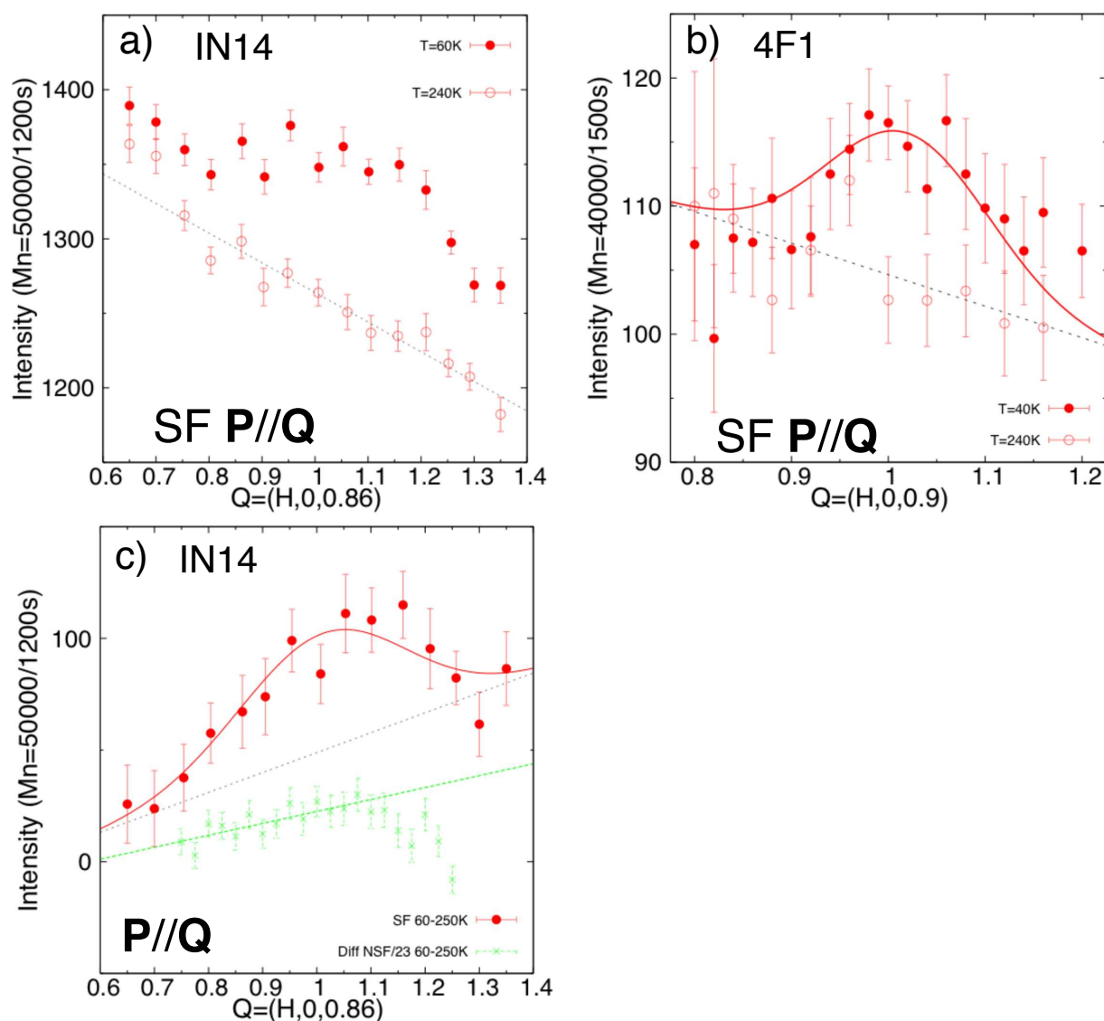
FIG. 6.8: Etude du cas où l'ordre est faiblement corrélé (en neutrons polarisés pour k_i=1.55\text{\AA}^{-1} ) : a) Intensité SF le long de la direction (\text{H}, 0, 9) autour de \text{H}=1 pour \text{P//Q} à T=60\text{K} (points rouges fermés) et T=250\text{K} (points rouges ouverts) sur le spectromètre froid IN14. b) Même chose qu'en a) sur le spectromètre froid 4F1 pour T=40\text{K} et T=250\text{K} . c) Différence entre les intensités SF (en points rouges fermés) et NSF (en points verts) mesurées le long de la direction (\text{H}, 0, 9) autour de \text{H}=1 pour \text{P//Q} à T=60\text{K} et T=250\text{K} . Dans le cas du canal NSF, la différence a été divisée par le rapport de flipping R où R=23 sur le spectromètre IN14 pour \text{P//Q} .
