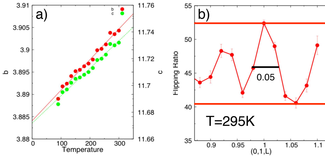
FIG. 5.4: a) Evolution du paramètre cristallin c en fonction de la température à k_i=2.662\text{\AA}^{-1} b) Evolution du rapport de flipping le long de la direction (0, 1, L) à T=295\text{K} pour l'échantillon A.
