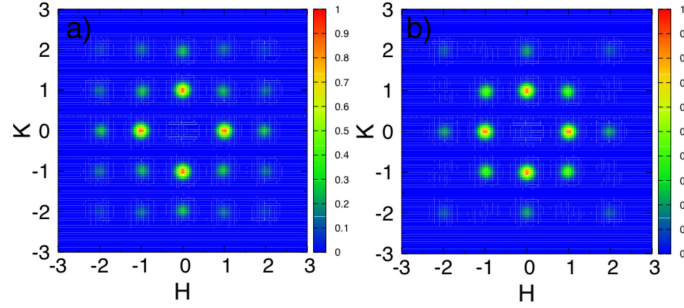
FIG. 4.6: Carte de l'intensité magnétique dans le plan de l'espace réciproque (H, K) pour a) la distribution de spin compatible avec la phase CC - \theta_{II} , b) pour la phase CC - \theta_{II} . Dans les deux cas, on a tenu compte des deux domaines suivant Eq.4.8
