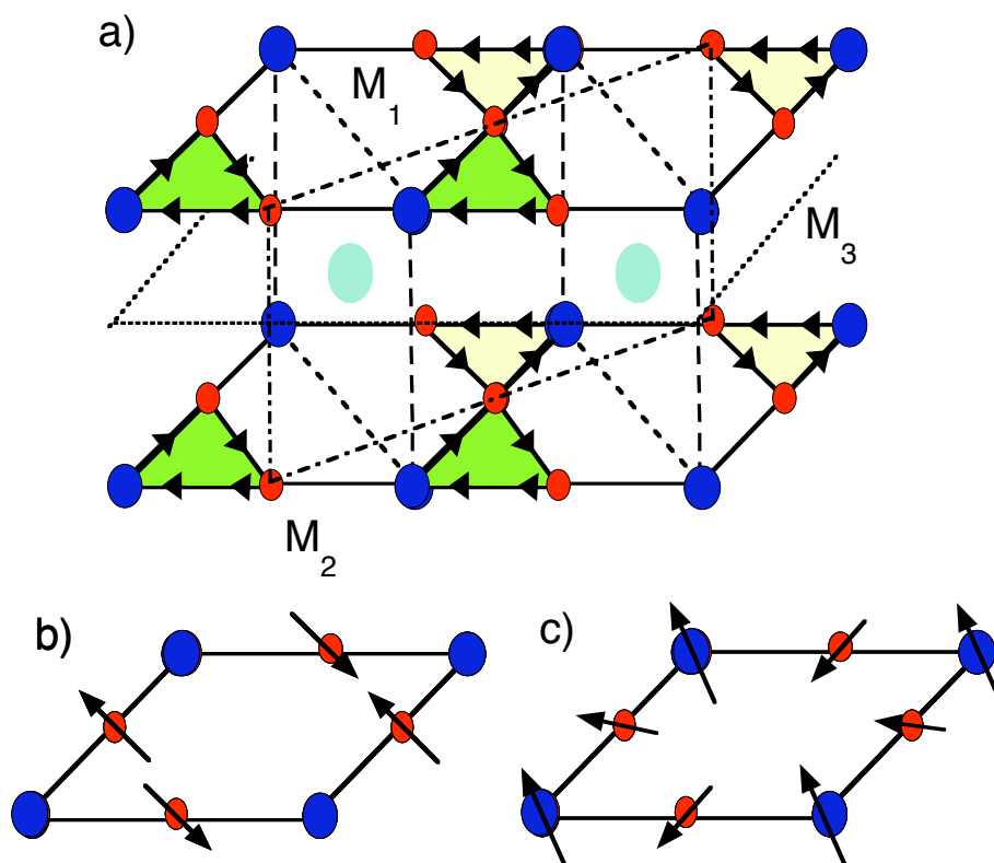
FIG. 5.10: a) Schéma du biplan CuO 2 du composé YBa 2 Cu 3 O 6+x en présence de la phase CC-\theta_{II} , en bleu les atomes de cuivre, en rouge les atomes de d'oxygène et en vert l'atome d'yttrium. (M 1 ), (M 2 ) et (M 3 ) sont trois plans de symétrie de la distribution de courant de la phase CC-\theta_{II} . b) Modèle de spin dans le plan CuO 2 alternatif à la phase CC-\theta_{II} ayant la symétrie compatible avec nos mesures. c) Ordre de spin induit par le couplage spin-orbite accompagnant la phase CC-\theta_{II} d'après [227].
