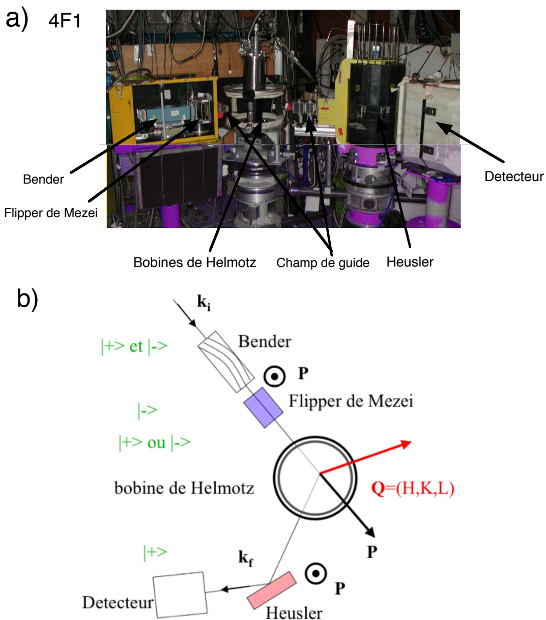
FIG. 2.5: Montage de neutrons polarisés sur 4F1 : a) la polarisation sur k_i est réalisée par un bender (en bleu) suivi d'un flipper de Mezei. La polarisation au niveau de l'échantillon est contrôlée par des bobines de Helmotz. L'analyse de polarisation est réalisée par un cristal de Heusler. b) Même chose que sur a), on reporte en plus l'état de polarisation du neutron ( |+\rangle et |-\rangle ) par rapport à la polarisation P des neutrons
