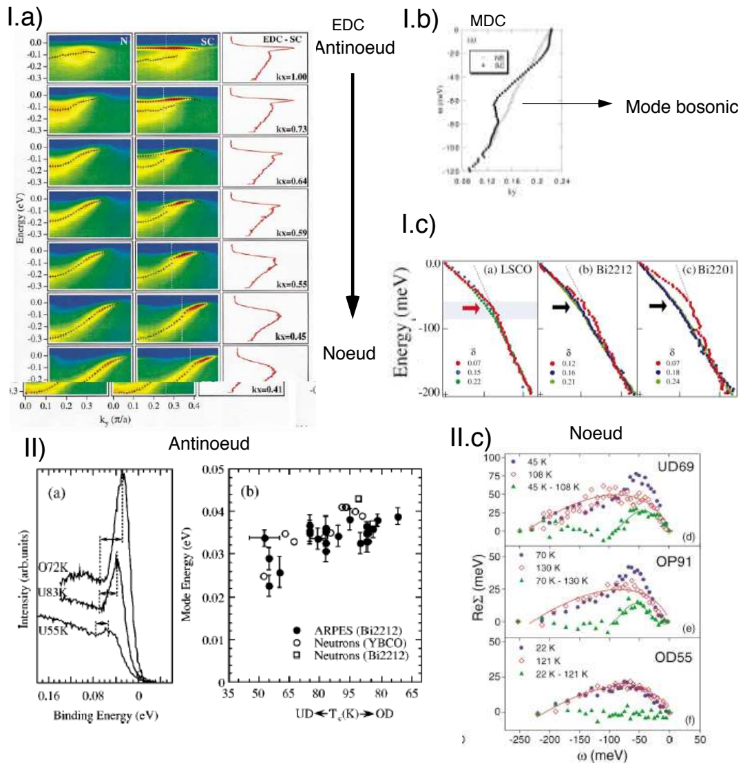
FIG. 1.11: I) a) D'après [130] : Intensité ARPES mesurée dans la phase normale ( T=140K ) et dans l'état supraconducteur ( T=40K ) pour un échantillon de Bi-2212 de T_c=89K le long de k_y pour différentes valeurs de k_x . Le panneau le plus haut correspond à un point se trouvant près du point nodal et le panneau le plus bas correspond à un point se trouvant près du point anti-nodal (AN). b) Dispersion MDC dans l'état supraconducteur et la phase normale pour un échantillon de dopage optimal de Bi-2212 de T_c=90K k_y (en unité de \pi/a ) et pour k_x=0.59\pi/a . c) Dispersion MDC pour différents dopages et différents cuprates. II) D'après [132] : Spectres d'ARPES pour le composé Bi-2212 au vecteur d'onde (\pi, 0) pour différents dopages, les flèches indiquent comment \Omega est déterminé à partir de ce spectre. À droite, comparaison entre la dépendance en dopage du mode \Omega déduite des mesures d'ARPES et de la position en énergie du pic de résonance magnétique. b) D'après [140], partie réelle de la self énergie en fonction de l'énergie dans les phase supraconductrice, normale ainsi que la différence des deux pour trois échantillons : un sous-dopé ( T_c=69K , un de dopage optimal ( T_c=91K ) et un surdopé ( T_c=55K ).
